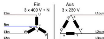
SPT: Y-Δ Anschluss
